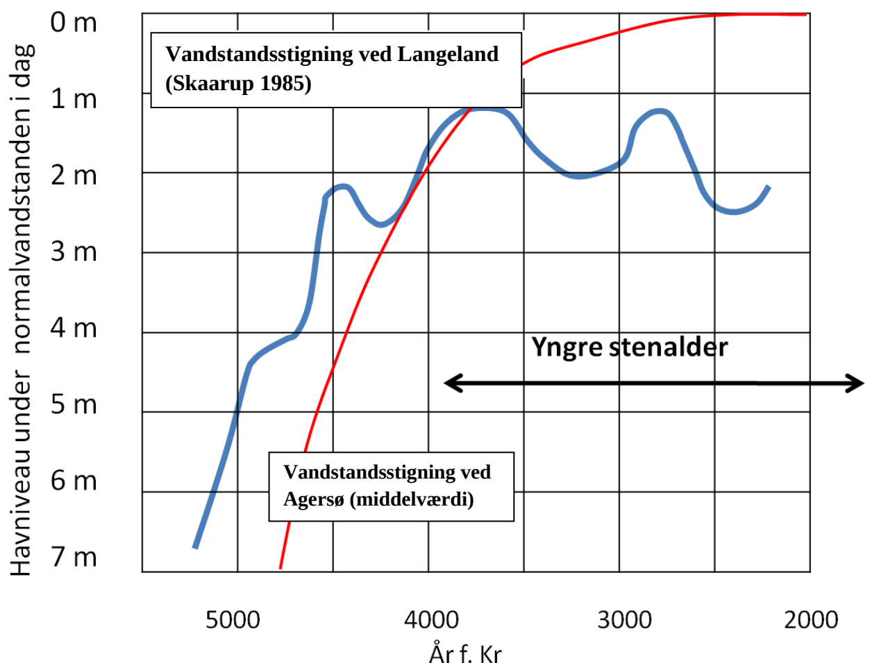
Figur 29. Havstigningen ved Agersø (rød kurve) fundet som middelværdi mellem målinger ved Langeland (Skårup 1985) og Vedbæk (Brinch Petersen 2006).
