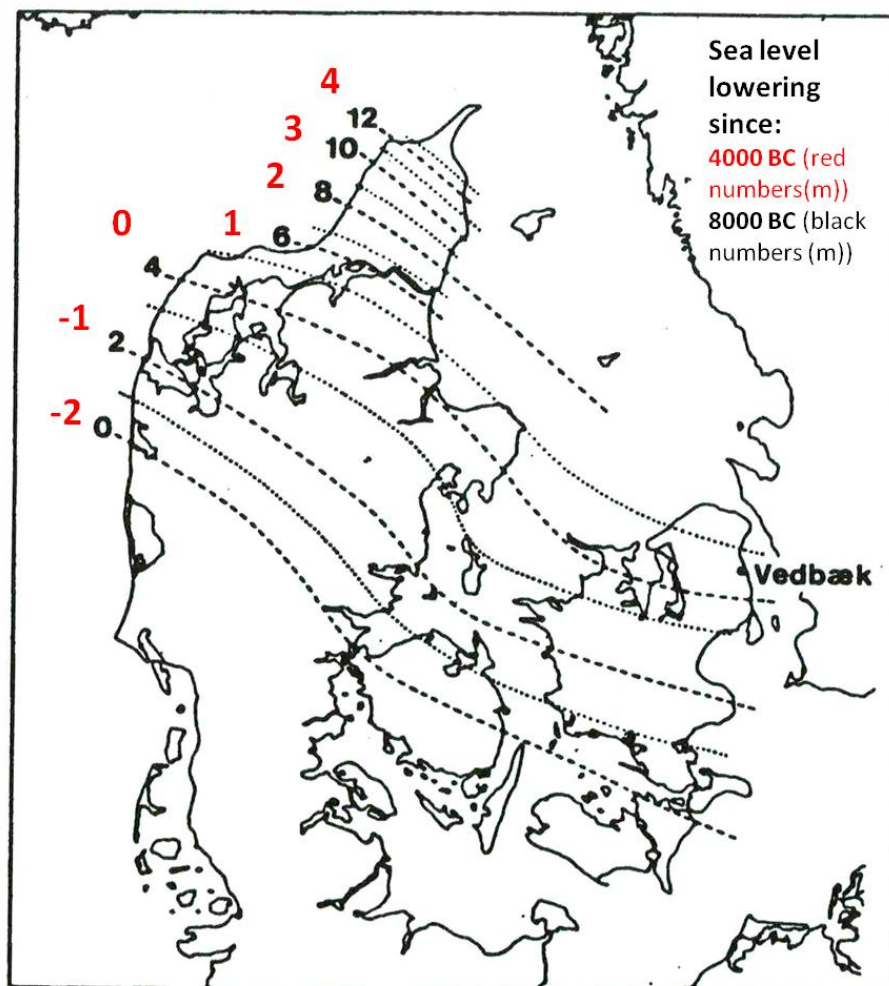
Figur 28. Vipningen af Danmark efter at istidsbræen har trukket sig tilbage. Kystlinien ved Agersø lå 2 m lavere ved yngre stenalders start (4.000 f.Kr.) [efter Mertz 1924].
