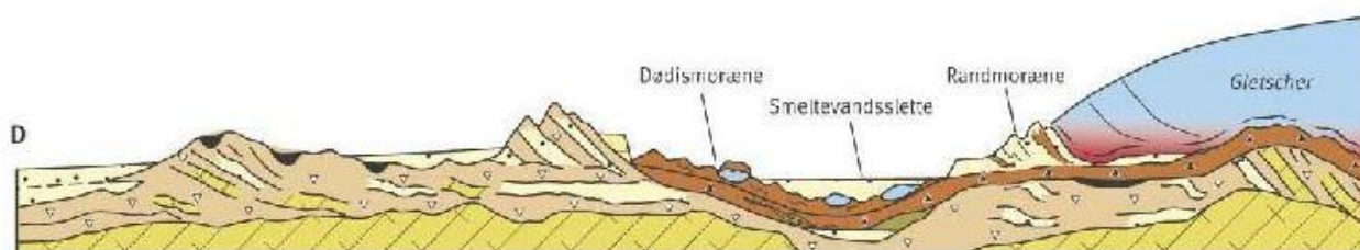
Figur 26. Profil af et typisk morænelandskab med isbræen til højre. Isen efterlader morænebakker og dødishuller. [Houmark-Nielsen et al. 2005, p.12].
